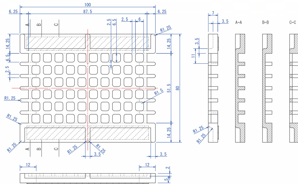
歩車道一体型 高上げタイプ
